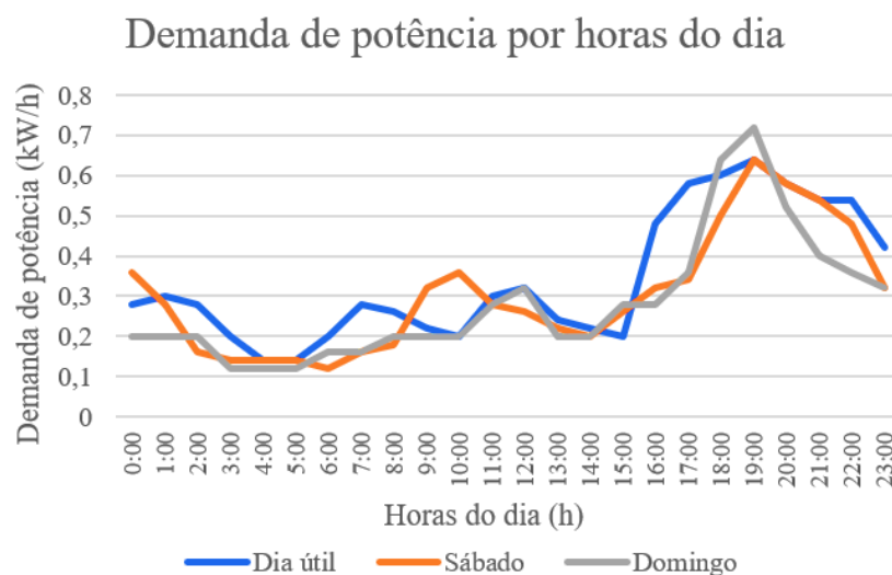
Fig.2 Demanda de potência dos dias típicos (Adaptado de [10])
