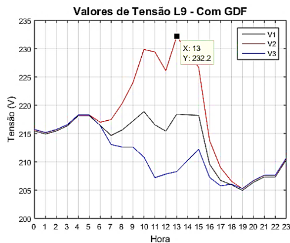
Fig.6 Tensão no ponto L9 para dia útil típico de janeiro-Com GDF
