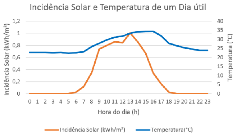
Fig.3 Incidência solar e temperatura de um dia de janeiro, INMET
