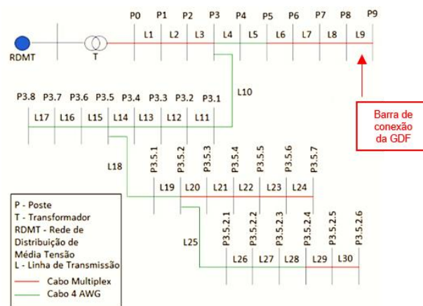
Fig.4 Diagrama da rede de distribuição do estudo de caso
