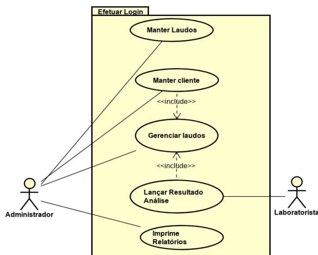
Fig.4 Diagrama de caso de uso
