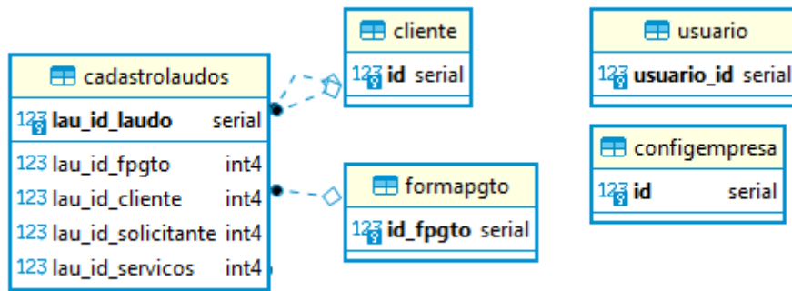
Fig.2 Diagrama de Entidade de Relacionamento
