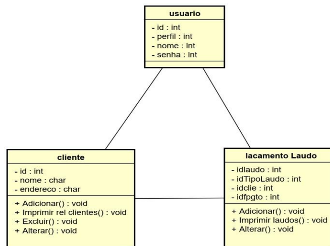
Fig.3 Diagrama de Classes
