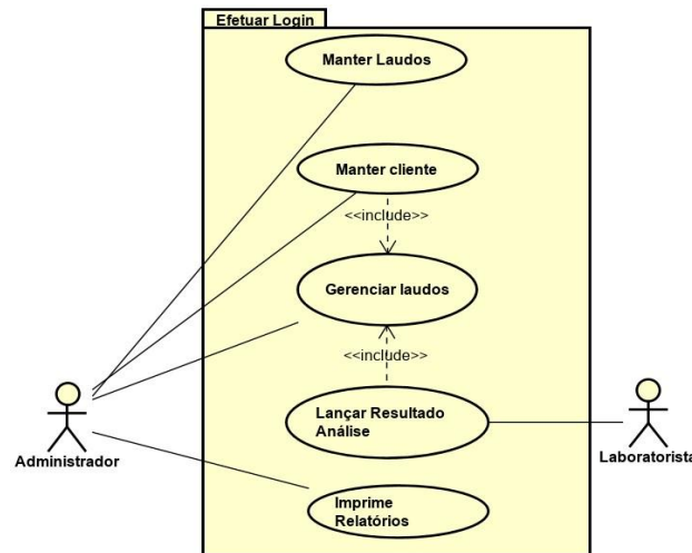
Fig.4 Diagrama de caso de uso
