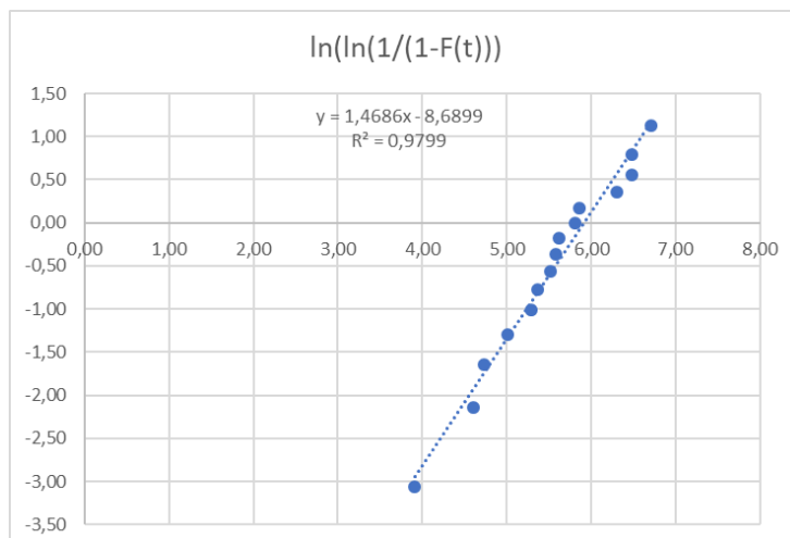
Fig. 1 Ecuación lineal de regresión para tiempos operativos de la cámara 3
