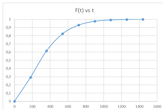
Fig.2 Densidad de la falla de la cámara 3
