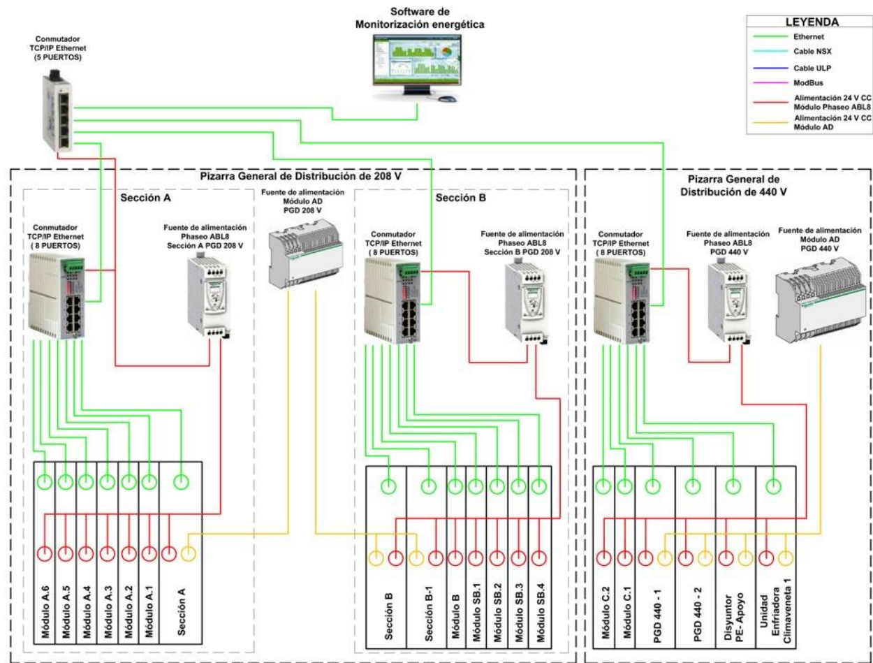
Fig.2 Arquitectura general de comunicación del sistema de monitorización de consumo de energía eléctrica en el Hotel Nacional de Cuba
