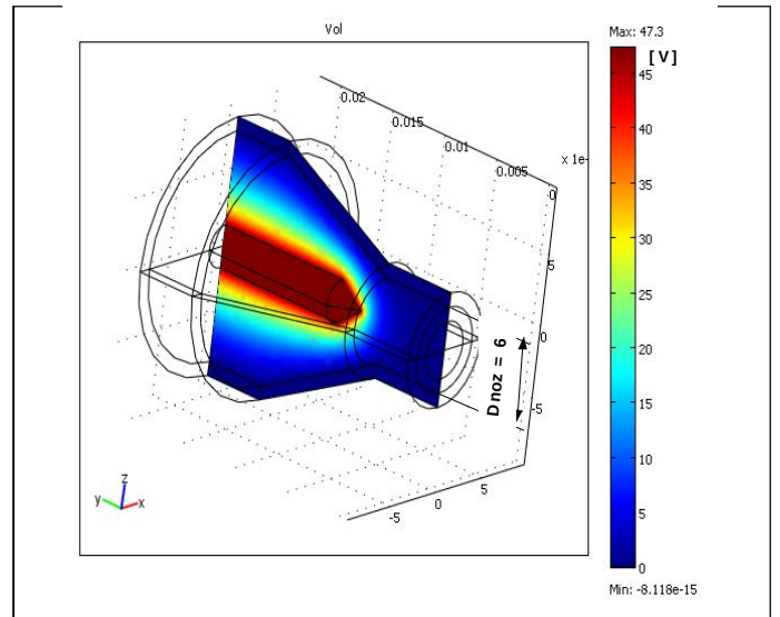
Fig. 5. Distribución del voltaje (V) en una sección del modelo 8 para t = 5 s.
