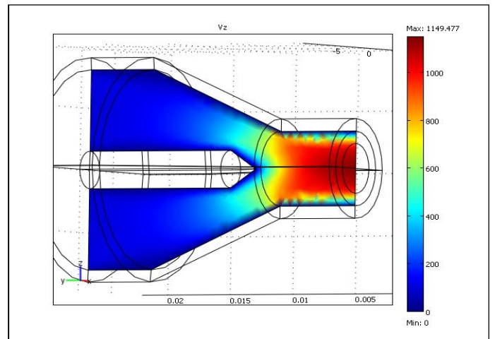
Fig. 7. Distribución de la velocidad del plasma (m/s) en una sección del modelo 8 para t = 5 s.
