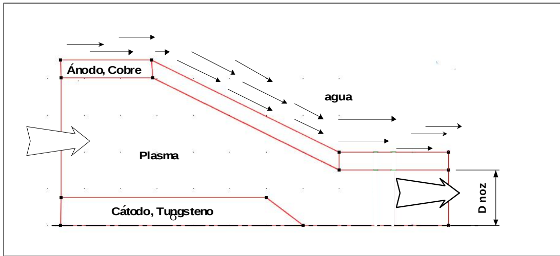
Fig. 2. Modelos de boquillas con D_{noz} = 6 \text{ mm} .
