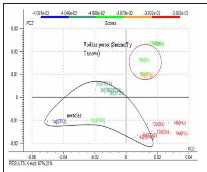
Fig. 5. Análisis de componentes principales a los espectros de los vodkas y mezclas después de aplicada la corrección de dispersión multiplicativa.
