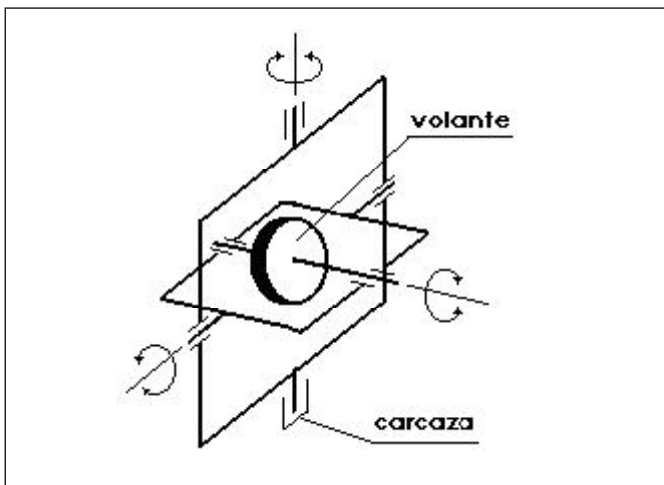
Fig. 2. Esquema de un giróscopo.
