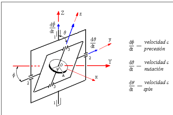
Fig. 3. Ángulos de Euler.
