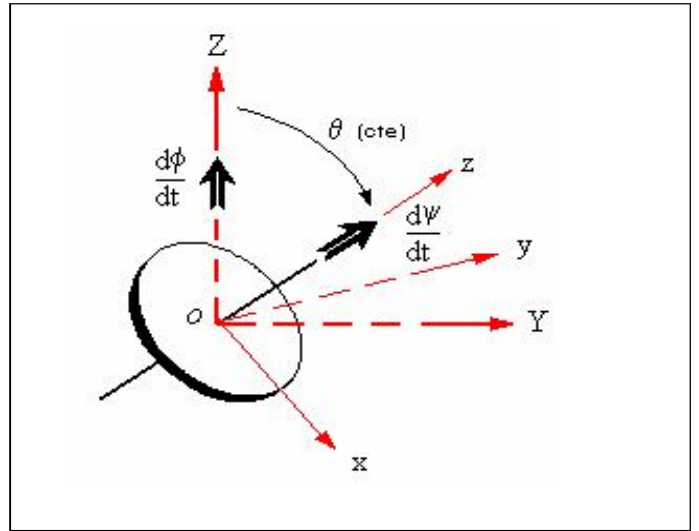
Fig. 5. Disco giroscópico.
