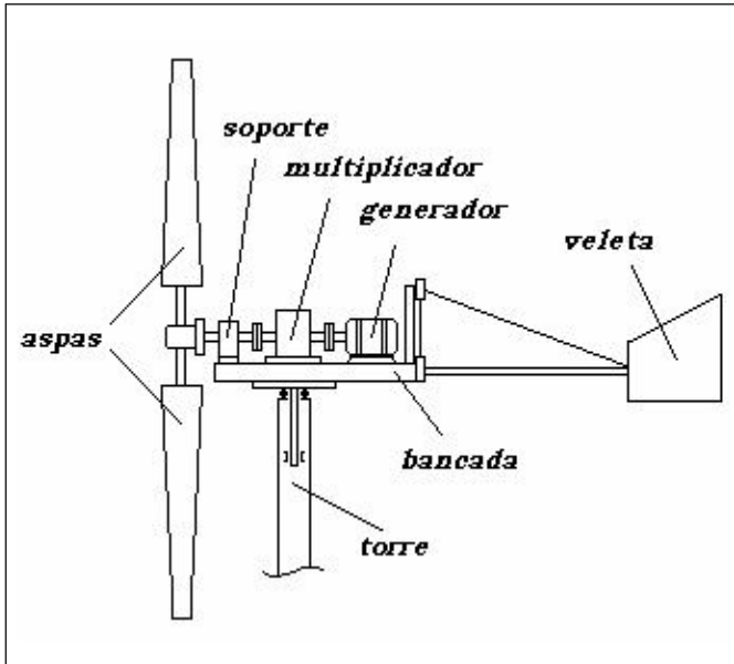
Fig. 1. Esquema elemental de un aerogenerador.
